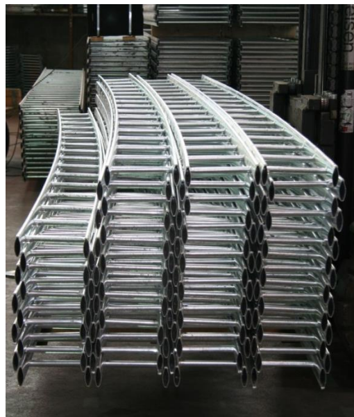
Fig.2: 300 mm kabelstige fremstillet til horizontal montage på tankanlæg med radius 72 m
